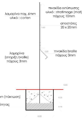
ΠΛΑΓΙΑ ΟΨΗ
