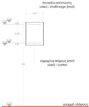
ΚΥΡΙΑ ΟΨΗ
