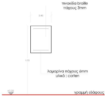
ΚΥΡΙΑ ΟΨΗ
